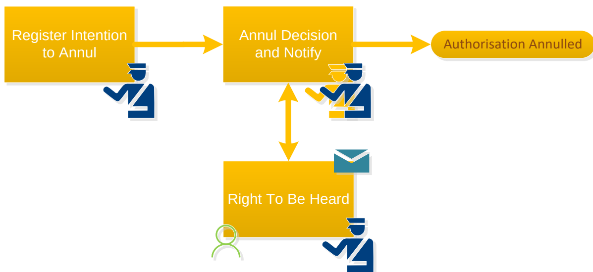
36. attēls. Anulēšanas procesa virslīmeņa pārskats
