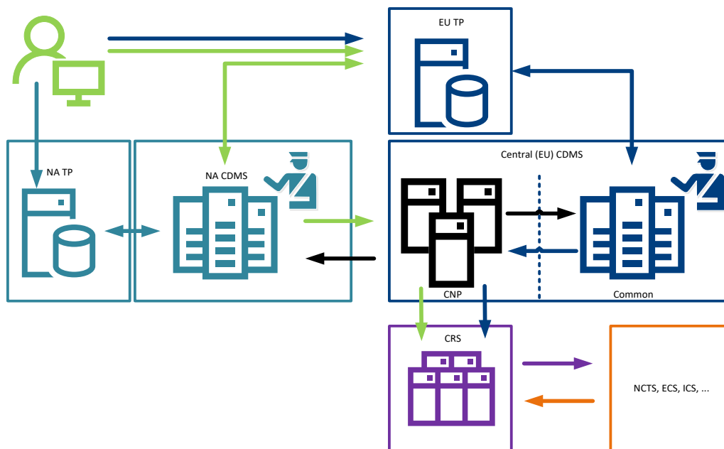
4. attēls. Muitas lēmumu sistēmas arhitektūras virslīmenis
